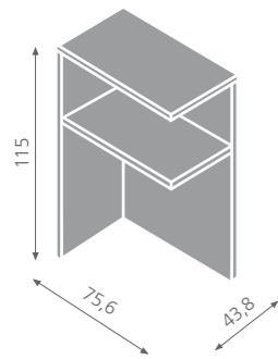
Contentore terminale / end cabinet / armoire final / abschluss schrank / armario terminal / терминальный модуль
